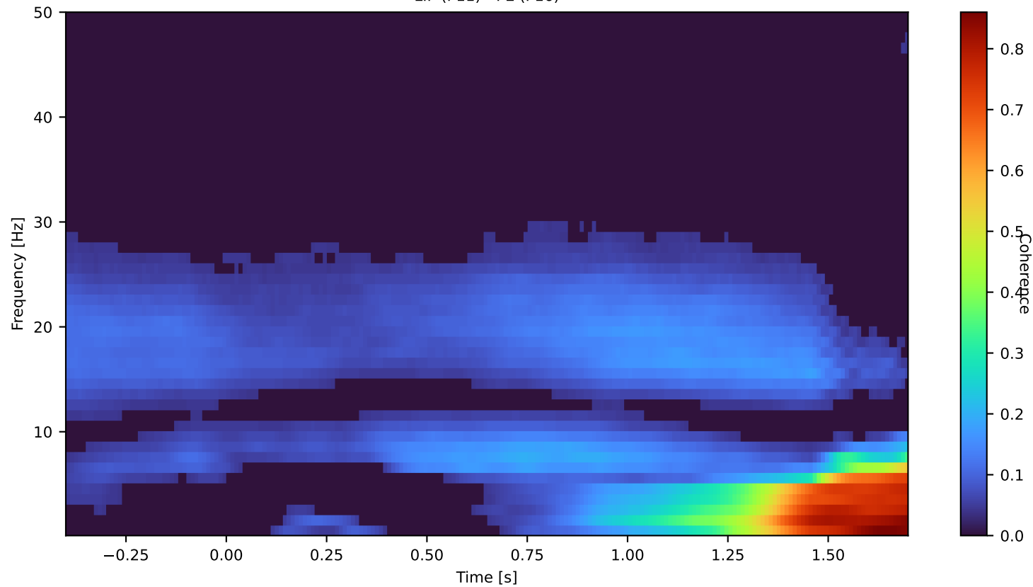
LIP (P11) - PE (P16)
